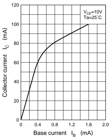
I_C - I_B
