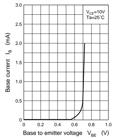
I_B - V_{BE}
